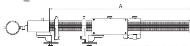
RANGE SPRING SYSTEM 20 MM. INSIDE/OUTSIDE CORSO UTILE PRECARICA 20 MM. INTERNO/ESTERNO
